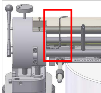
Abb. 11: Befestigen des Headshells
