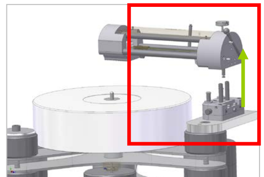
Abb.5: Aufsetzen des Tonarms
