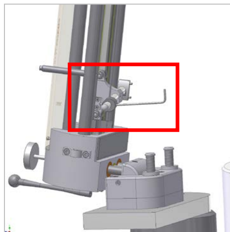
Abb.13: Befestigen der Gegengewichte
