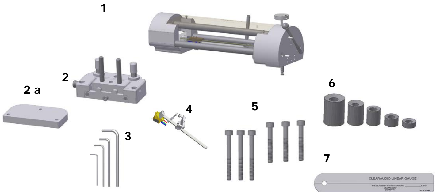
Abb.1: Lieferumfang
