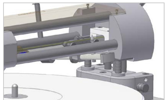
Abb. 9: Position nach Einsetzen des Headshells
