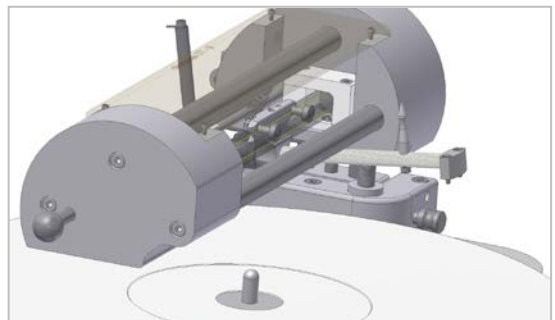
Abb. 6: Festschrauben der Höhenverstelleinheit
