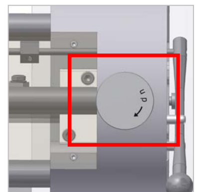
Abb.14: Höhenverstellung
