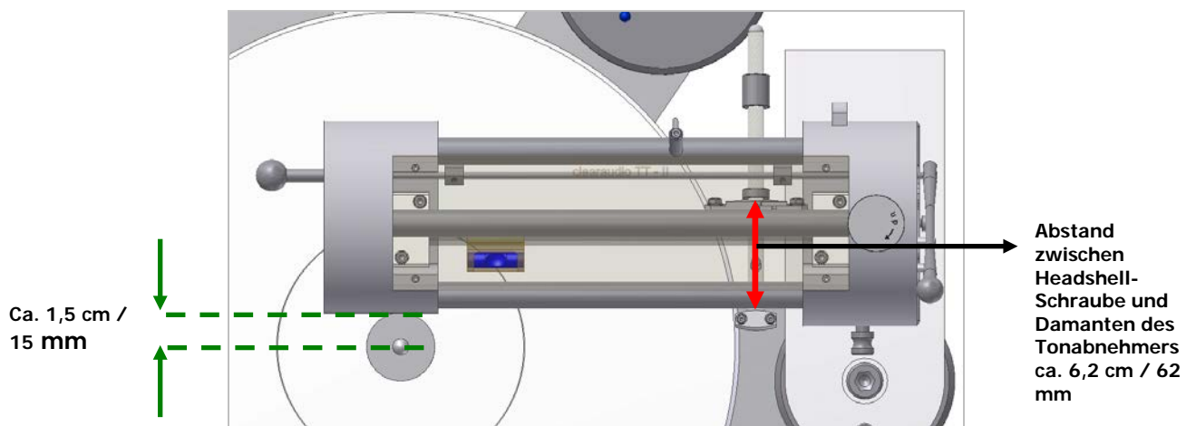
Abb. 10: Korrekte Position des Tonarms (Draufsicht)
