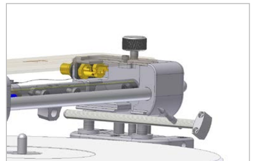
Abb. 7: Einsetzen des Headshells
