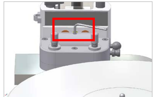
Abb. 6: Festschrauben der Basis
