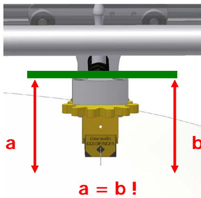
Abb.17: Azimuth - Einstellung
