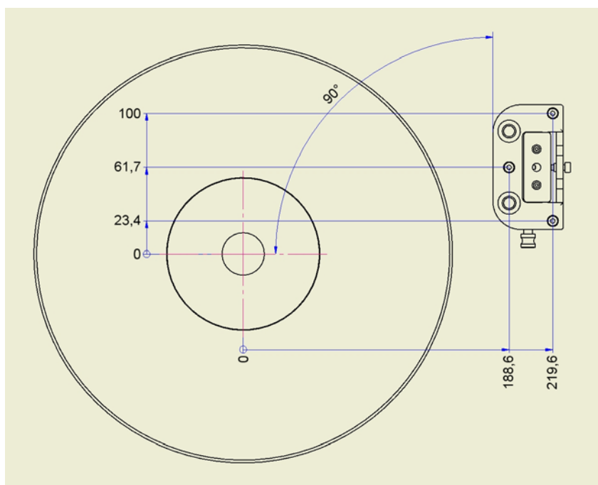
Abb.4: Bohrschablone
